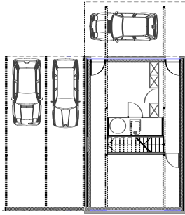
Grundriss UG
